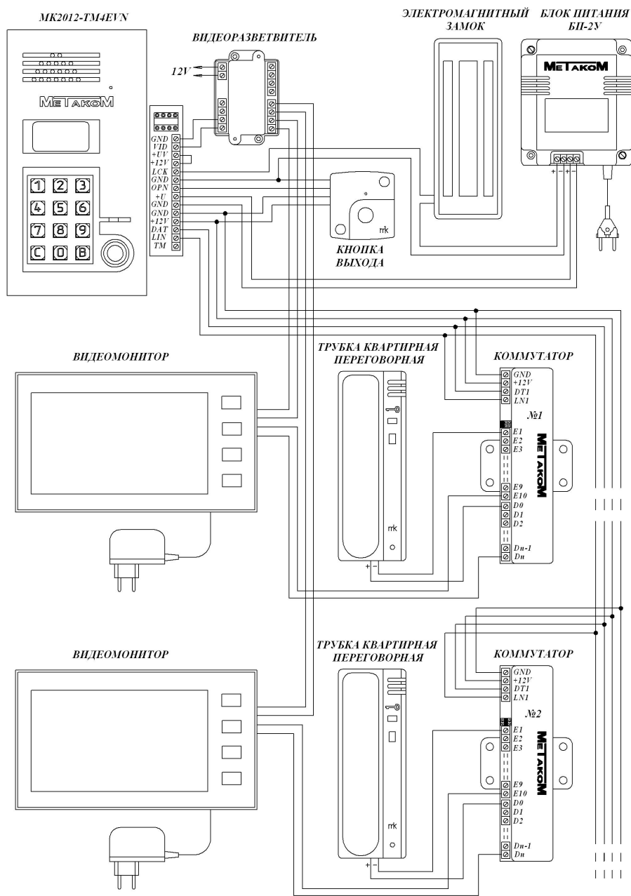
Рис. 2 Пример монтажа блока вызова МК2012-ТМ4ЕVN
