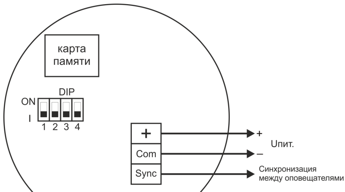
Рисунок 6 – Схема подключения РЗОР-Exd-10, РЗОР-Exd-20, РЗОР-Exd-30, РЗОР-Exd-50
