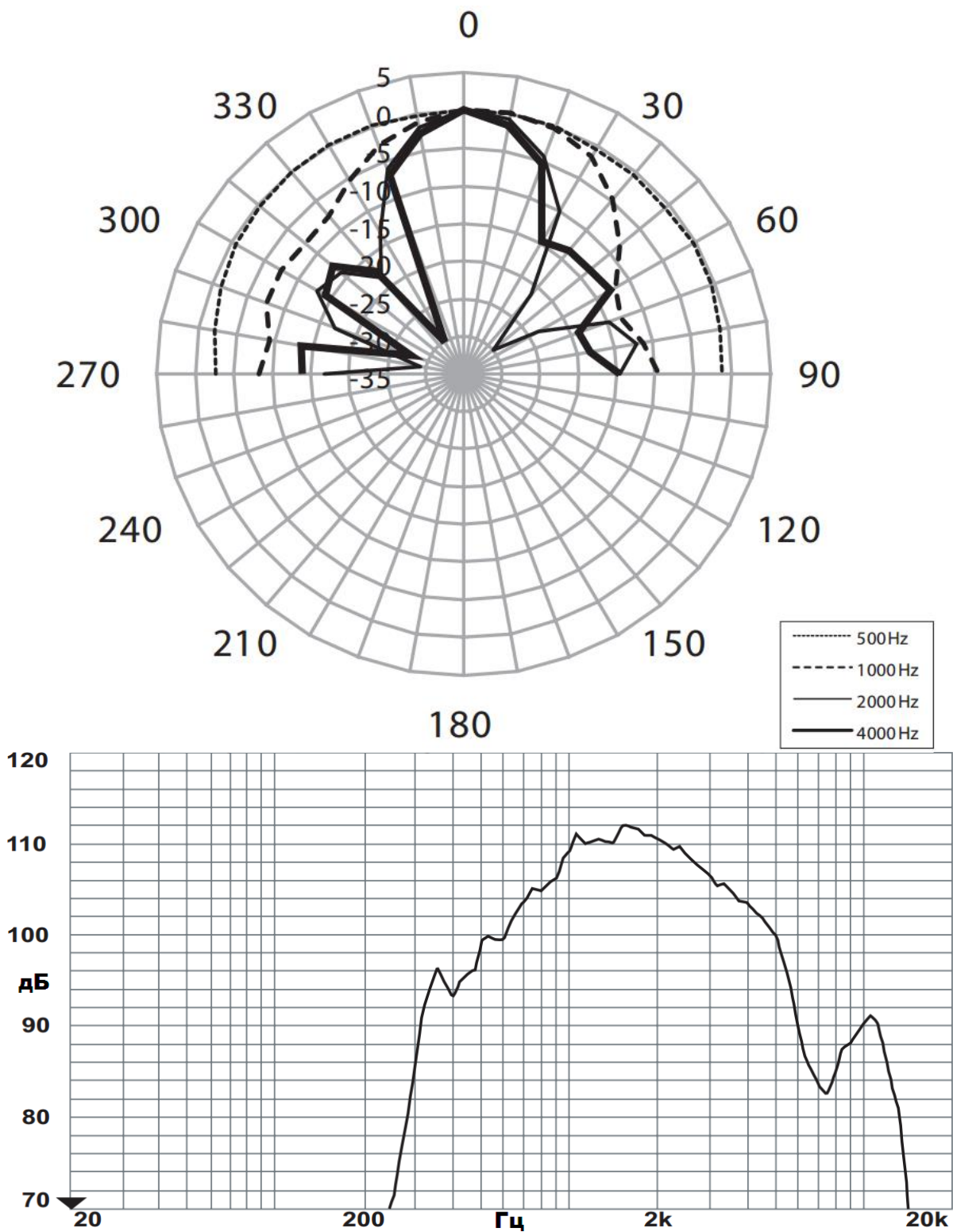
Рисунок 9 – Диаграмма направленности и амплитудно-частотная характеристика ГВП-Exd-10, P3OP-Exd-10, ГВП-Exd-20, P3OP-Exd-20
