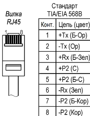
Рисунок 7 – Обжимка вилки RJ45 на кабель кат.5е
