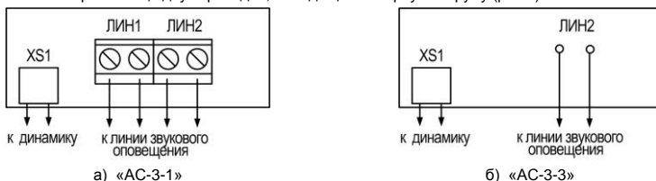
Рис.1 Платы «АС-3-1» и «АС-3-3». Схемы соединений
