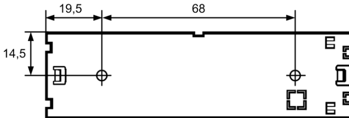
Рис.8 Основание. Присоединительные размеры
