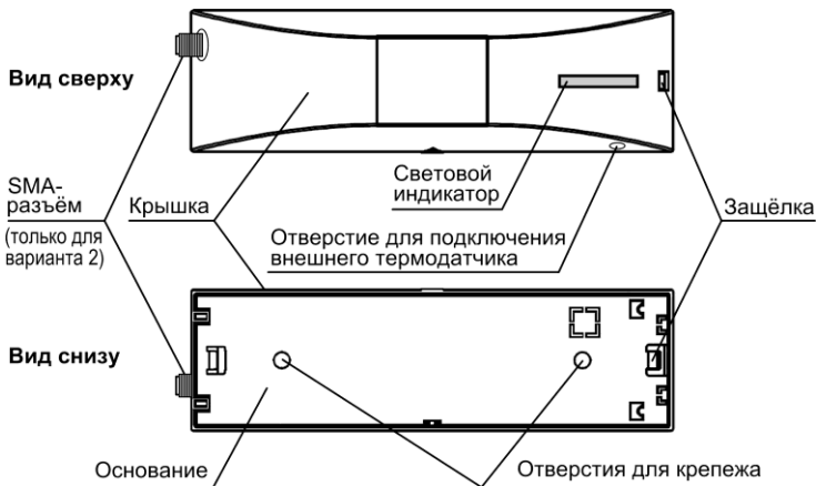
Рис.1 Конструкция сигнализатора. Вид сверху и снизу
