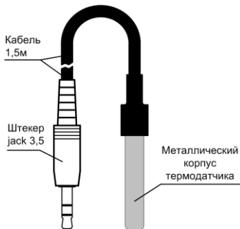
Рис.3 Внешний термодатчик
