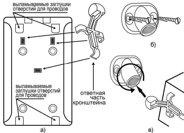
Рис.2 а) Вид на заднюю стенку извещателя; б) Крепление кронштейна; в) Схема соединения кронштейна и держателя
