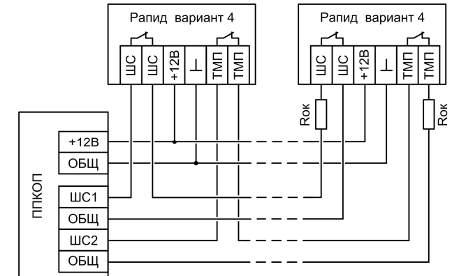
Рис.3 Схема подключения извещателей к ППКОП
