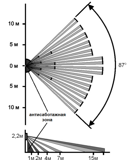
Рис.4 Диаграмма зоны обнаружения при установке извещателя на высоту 2,2 м и наклоне основания извещателя вниз (в вертикальной плоскости) на угол 12°
