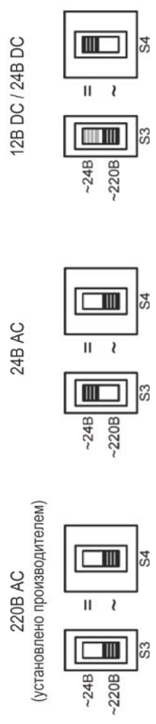
Рис.6 Схема переключения напряжения питания передатчика переключателями S3 и S4, расположенными на печатной плате (рис.1). Для вскрытия передатчика, необходимо отверткой через боковые пазы отогнуть защелки корпуса и выдвинуть крышку с печатной платой.
