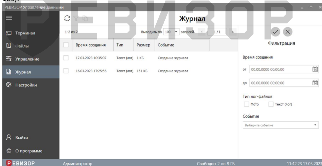
Рисунок 105 – Раздел Журнал
