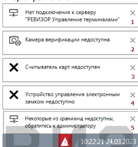
Рисунок 14 – Индикатор уведомлений
