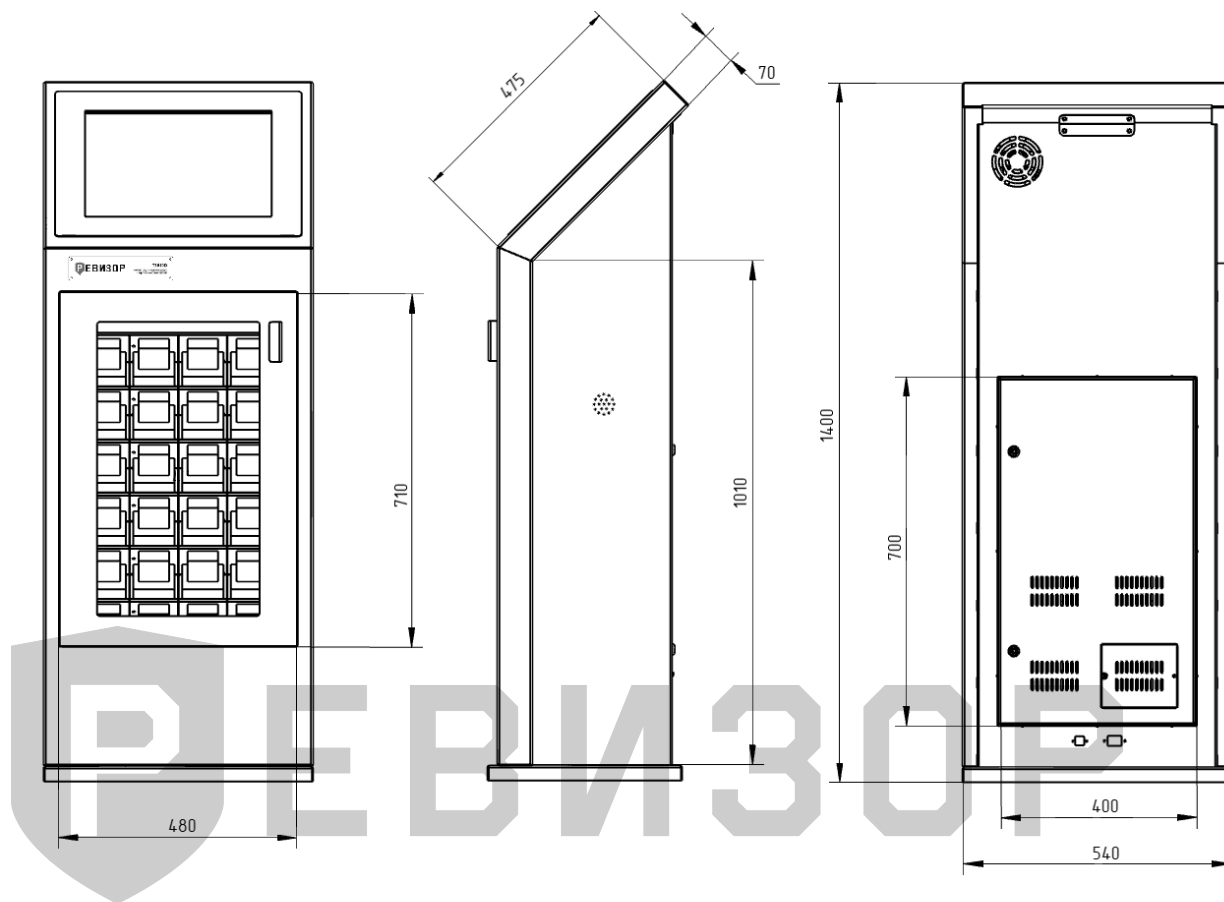
Рисунок 1 - Габаритные размеры терминала T20HDD/T24HDD/T28HDD
