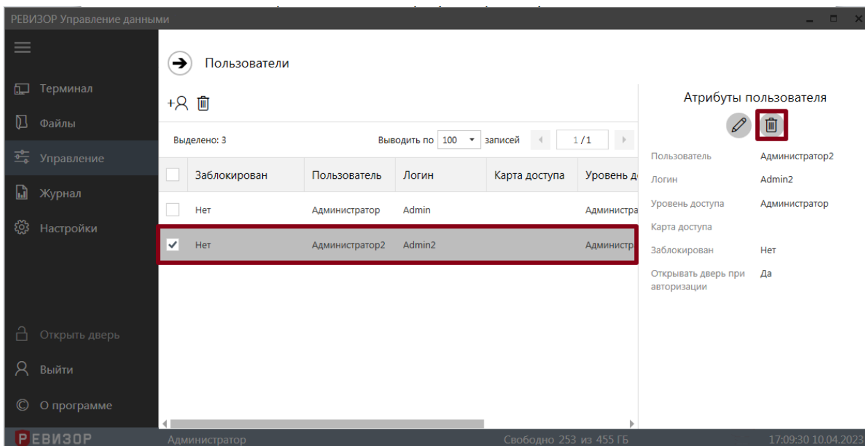
Рисунок 102 – Удаление «Пользователя»
