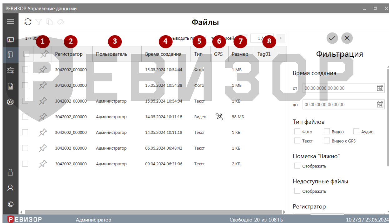
Рисунок 34 – Список «Файлов»
