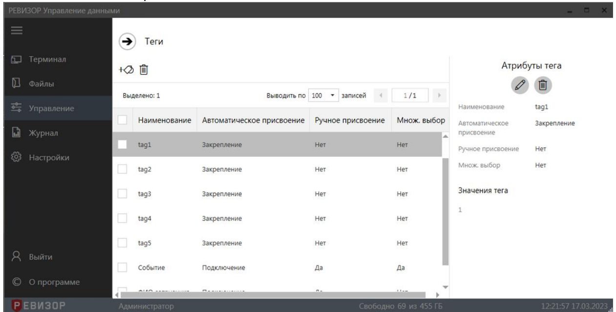
Рисунок 71 – Список «Тегов»
