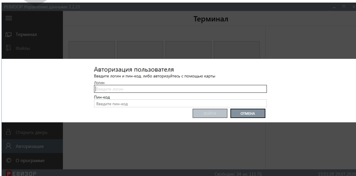
Рисунок 103 – Авторизация «Пользователя»
