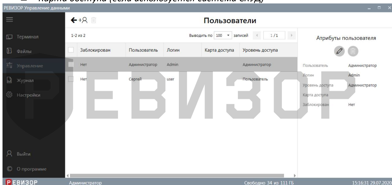
Рисунок 96 – Список «Пользователей»
