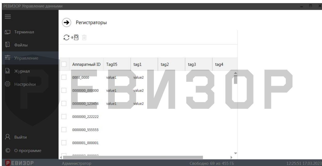
Рисунок 86 – Список «Регистраторов»
