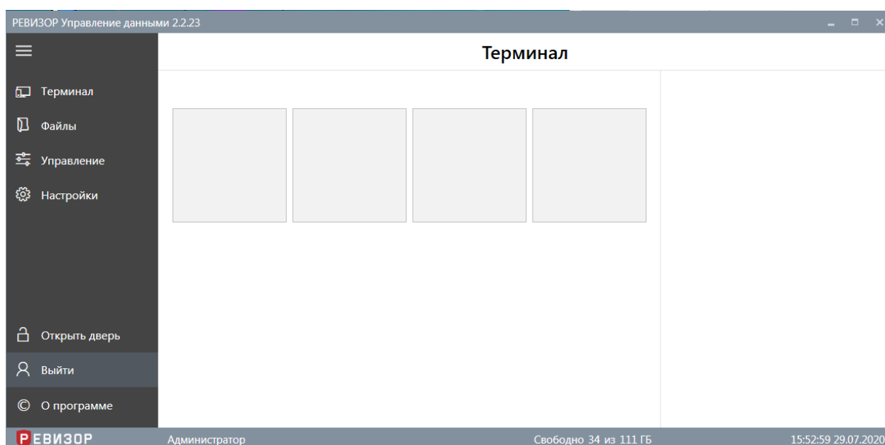
Рисунок 104 – Смена «Пользователя»
