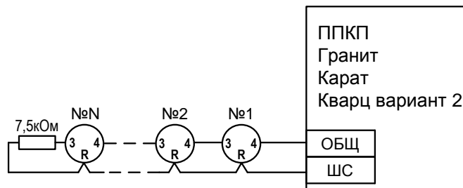
Рис.3 Схема подключения извещателей к ППКП «Гранит», «Карат» и «Кварц» вариант 2 производства ООО НПО «Сибирский Арсенал».
