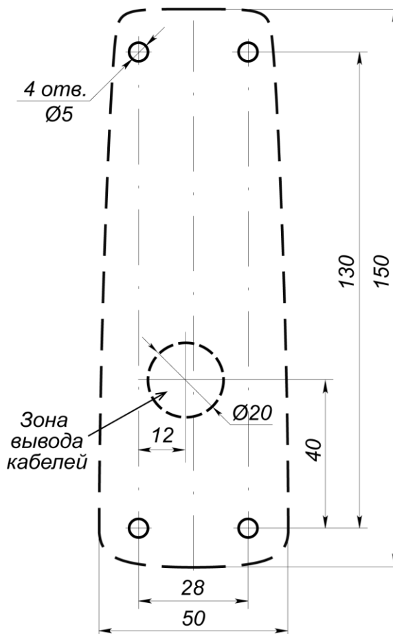
Рисунок 2. Разметка отверстий для установки контроллера (пунктиром показаны габариты корпуса контроллера)
