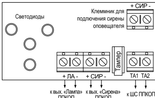
Рис.1 Схема подключения оповещателя к ППКОП
