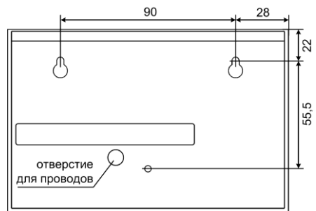
Рис.2 Основание. Присоединительные размеры
